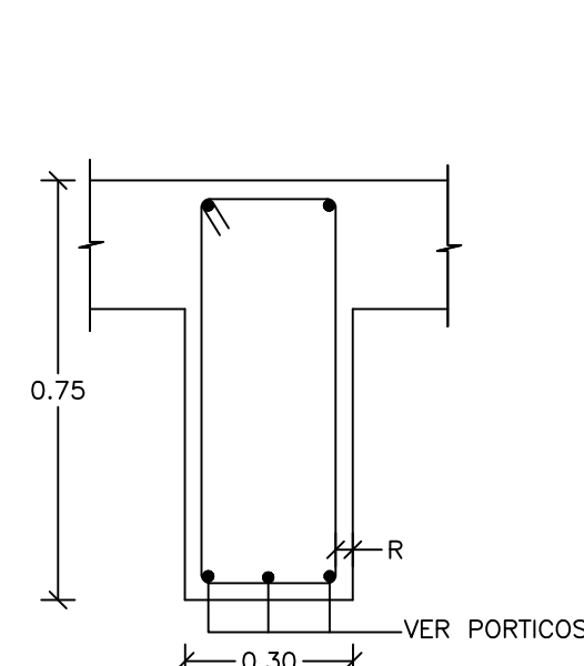
5 SECCION "P2" ES-10 ESC. 1:15
