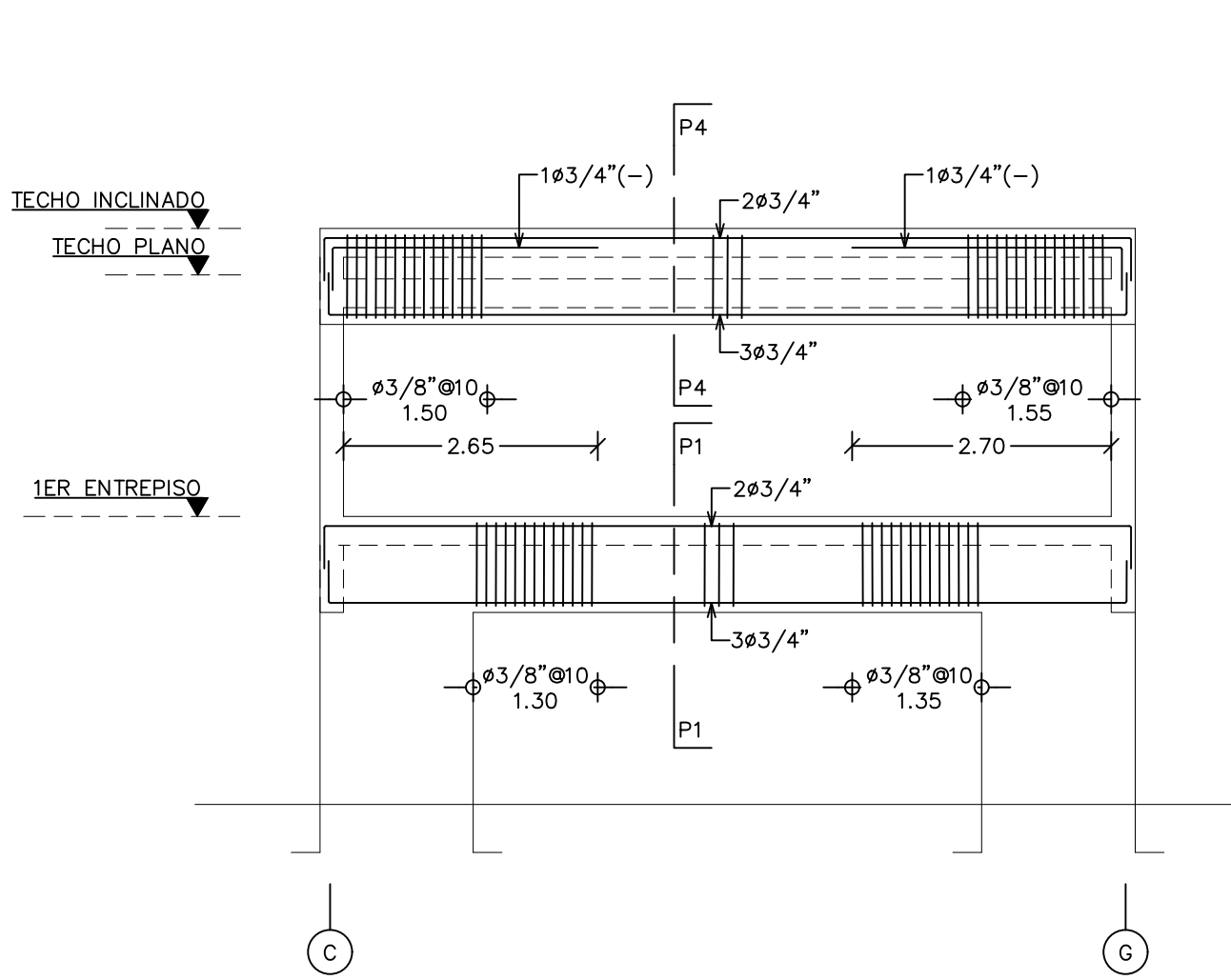
3 DETALLE PORTICO "10Y" ES-10 ESC. 1:75
