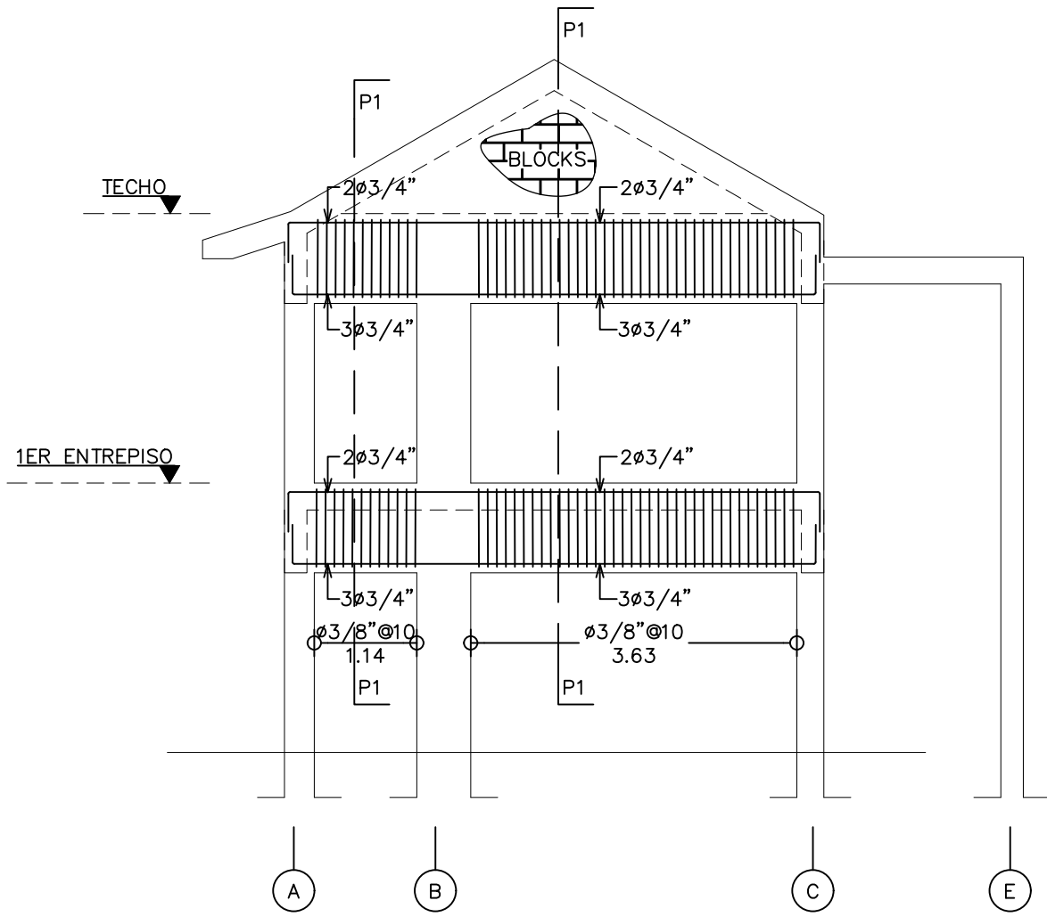
1 DETALLE PORTICO "8Y" ES-10 ESC. 1:75
