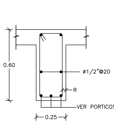
7 SECCION "P4" ES-10 ESC. 1:15
