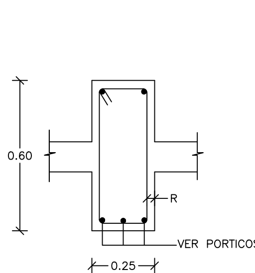
6 SECCION "P3" ES-10 ESC. 1:15
