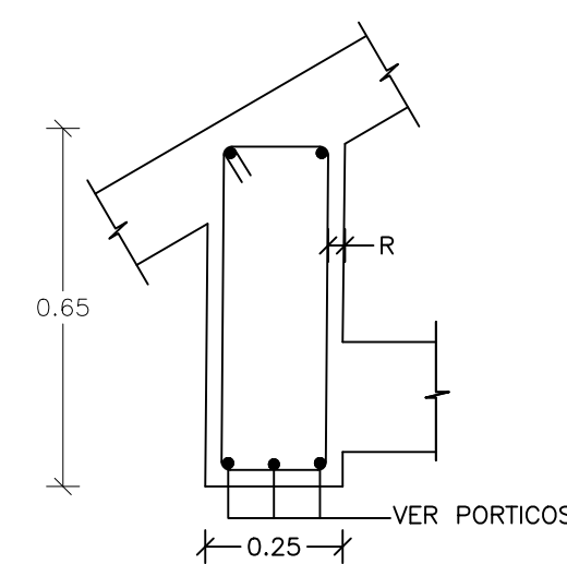
7 SECCION "P4" ES-10 ESC. 1:15
