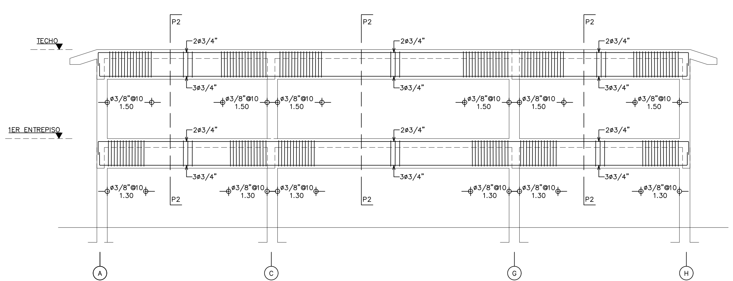
10 DETALLE PORTICO "12Y" ES-10 ESC. 1:75
