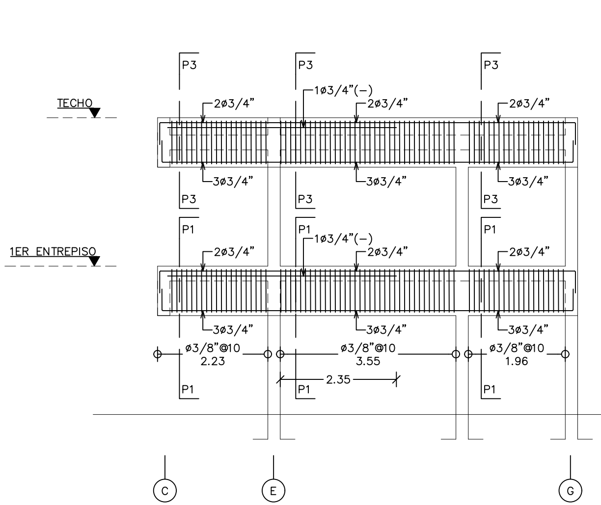
2 DETALLE PORTICO "9Y" ES-10 ESC. 1:75
