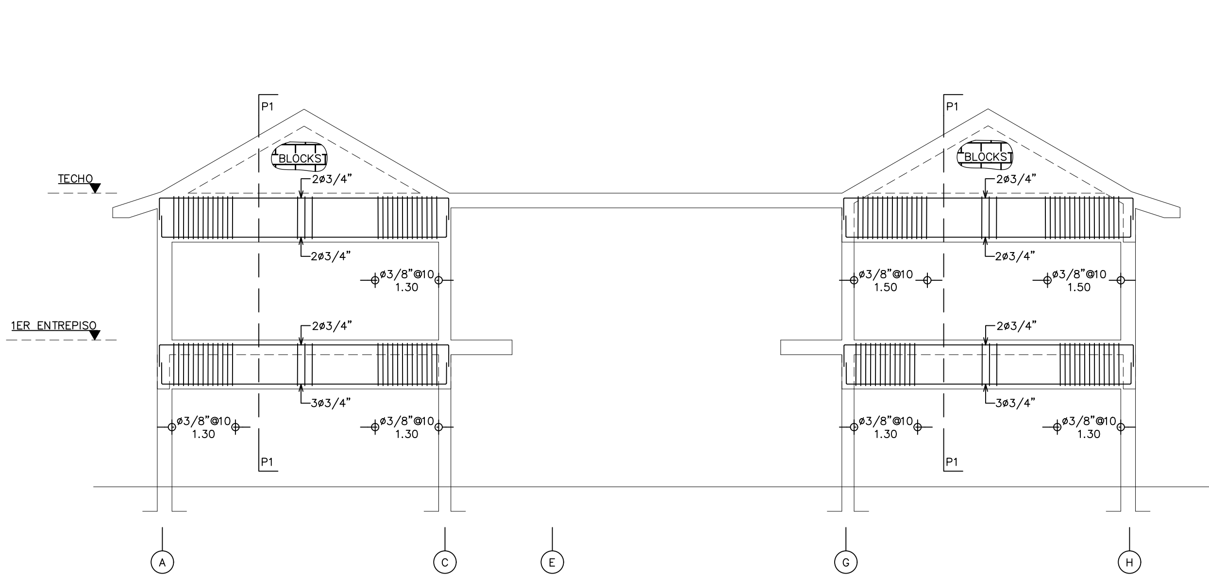
8 DETALLE PORTICO "10' Y" ES-10 ESC. 1:75
